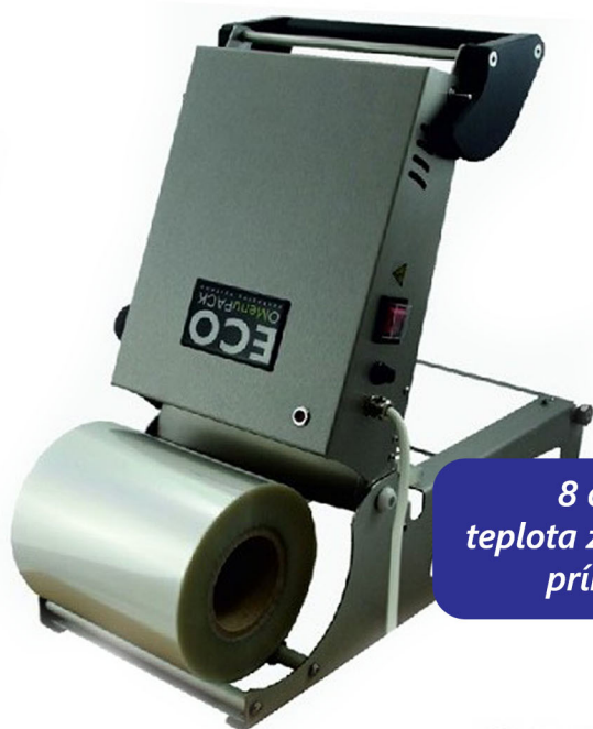
880801 Baliaci stroj na jedlo MP 1 x 1 ks na objednávku
